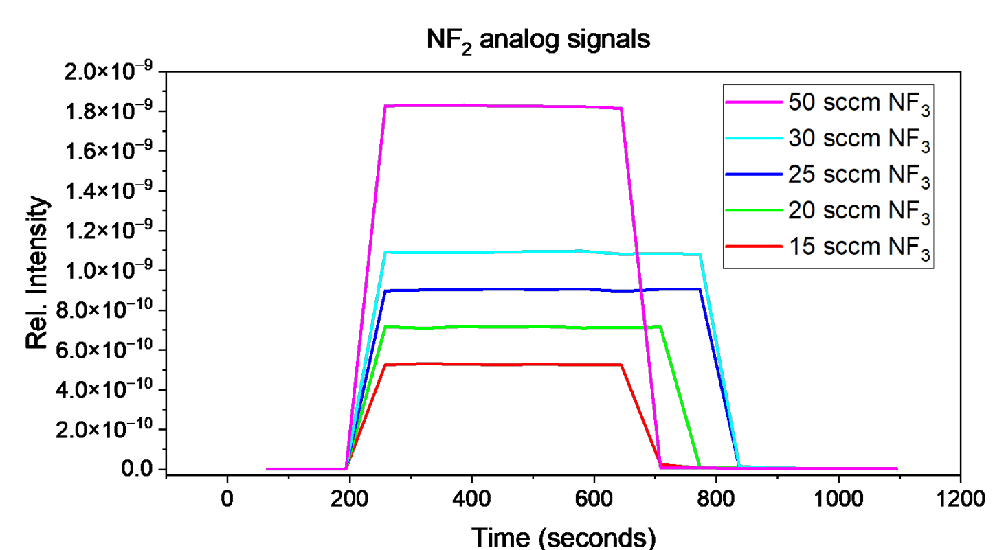
Abb. 3: Signalverlauf bei verschiedenen \text{NF}_3 -Konzentrationen im Trägergasstrom
